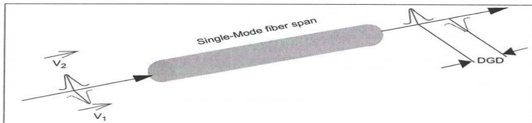
نمونه تاخیر نهائی بین دو لایه پولاریزاسیون
