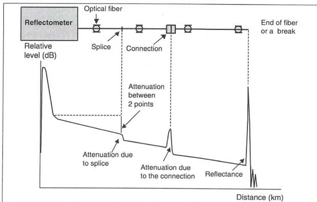
نمونه مسیر پخش برگشتی
